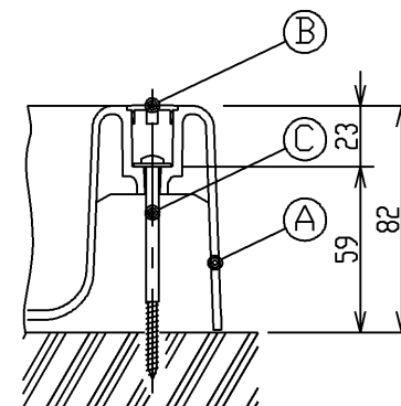
床固定部詳細(1:3)
